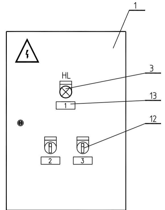
Вид спереди дверцы щита
