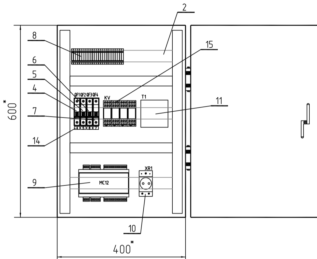
Вид задней стенки щита с расположением оборудования
