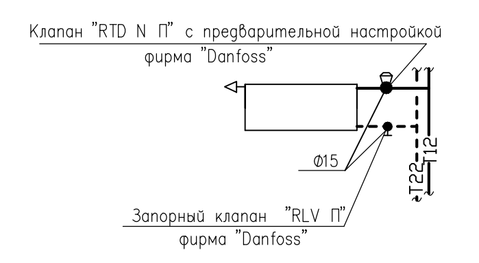
Распределительный узел
