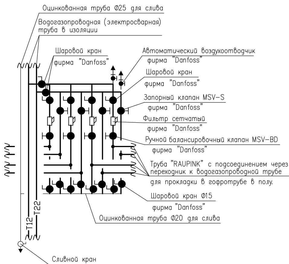
Распределительный узел
