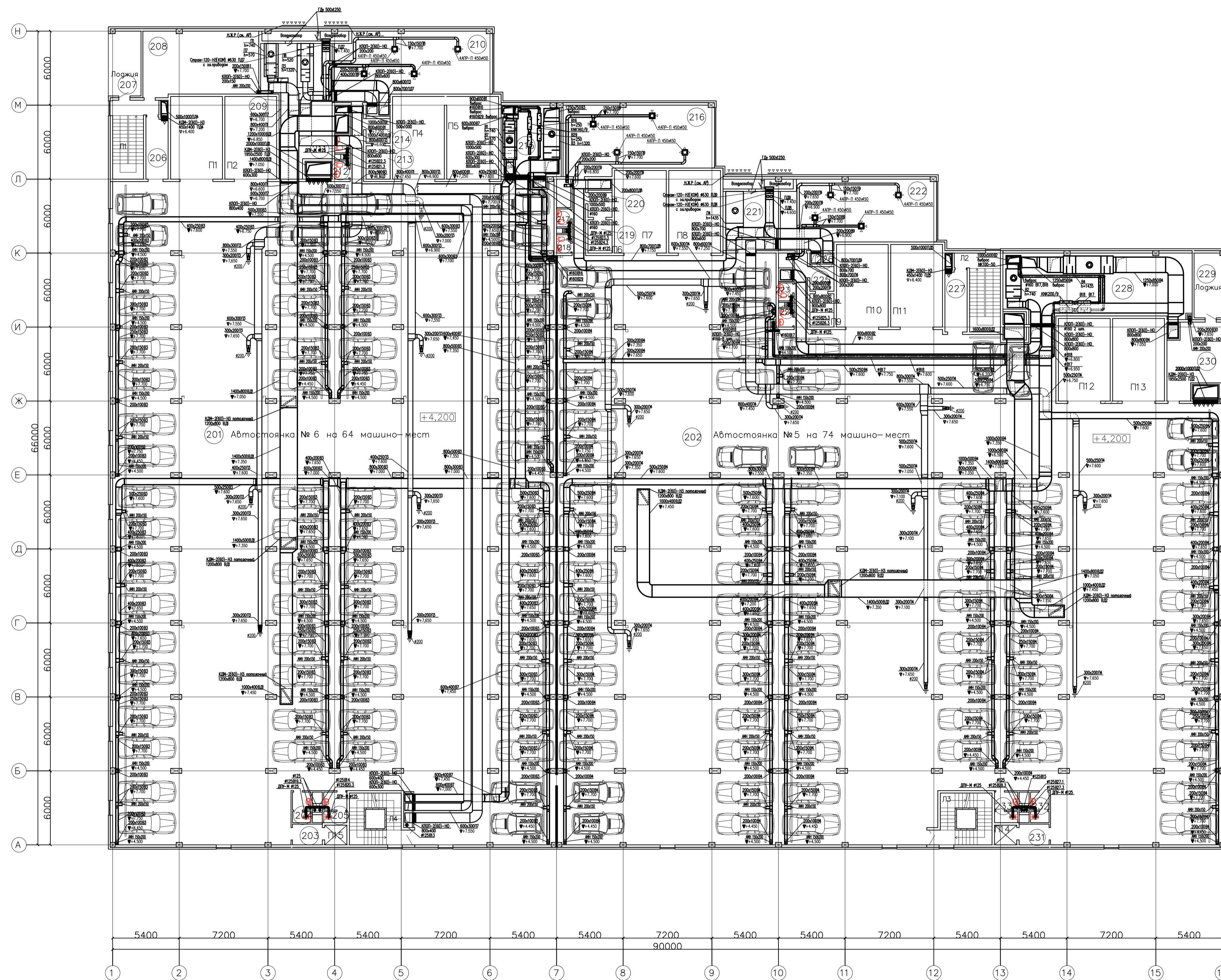
План 2-го этажа с системами вентиляции
