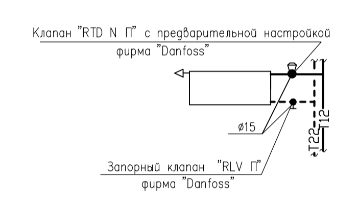
Распределительный узел
