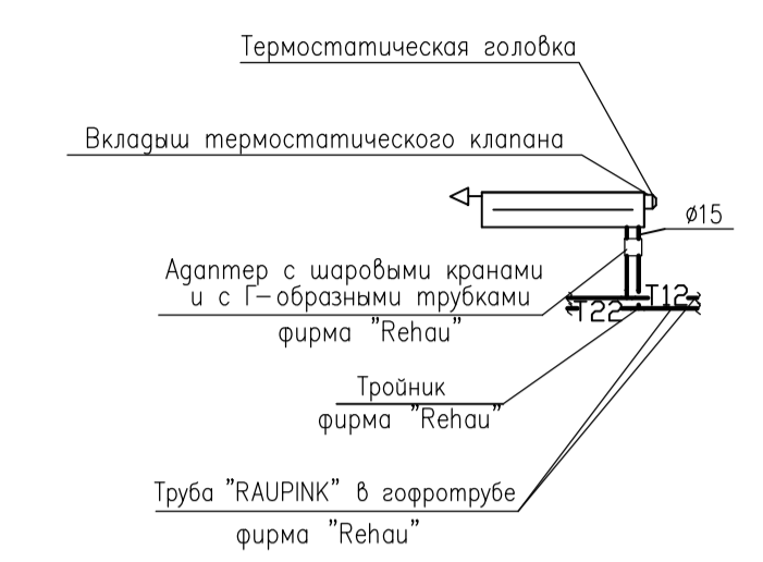
Подсоединение конвектора с нижней подводкой к системе отопления
