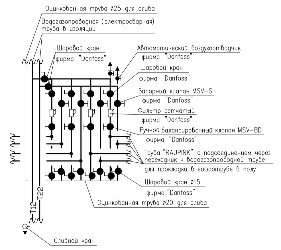
Распределительный узел
