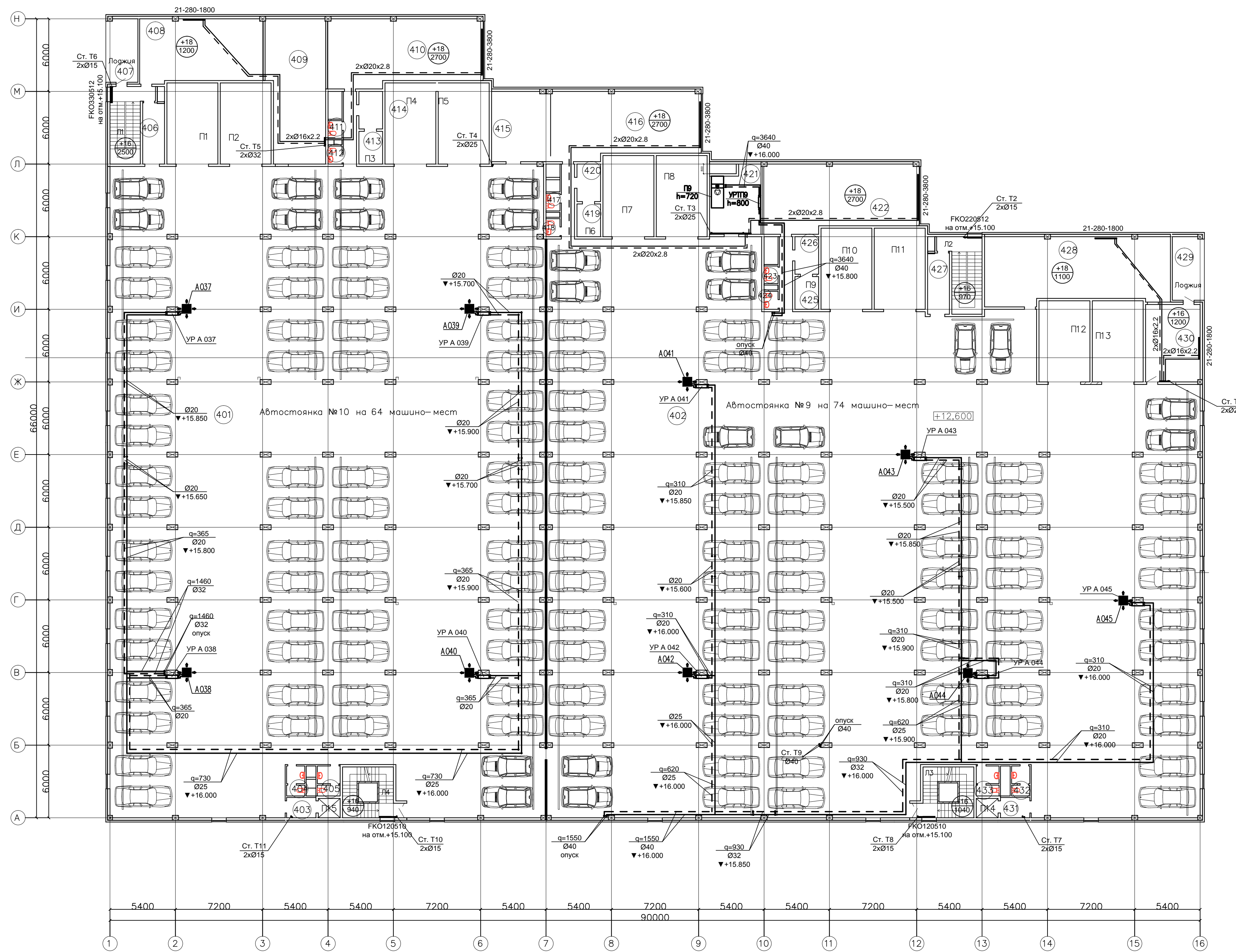
План 4-го этажа
