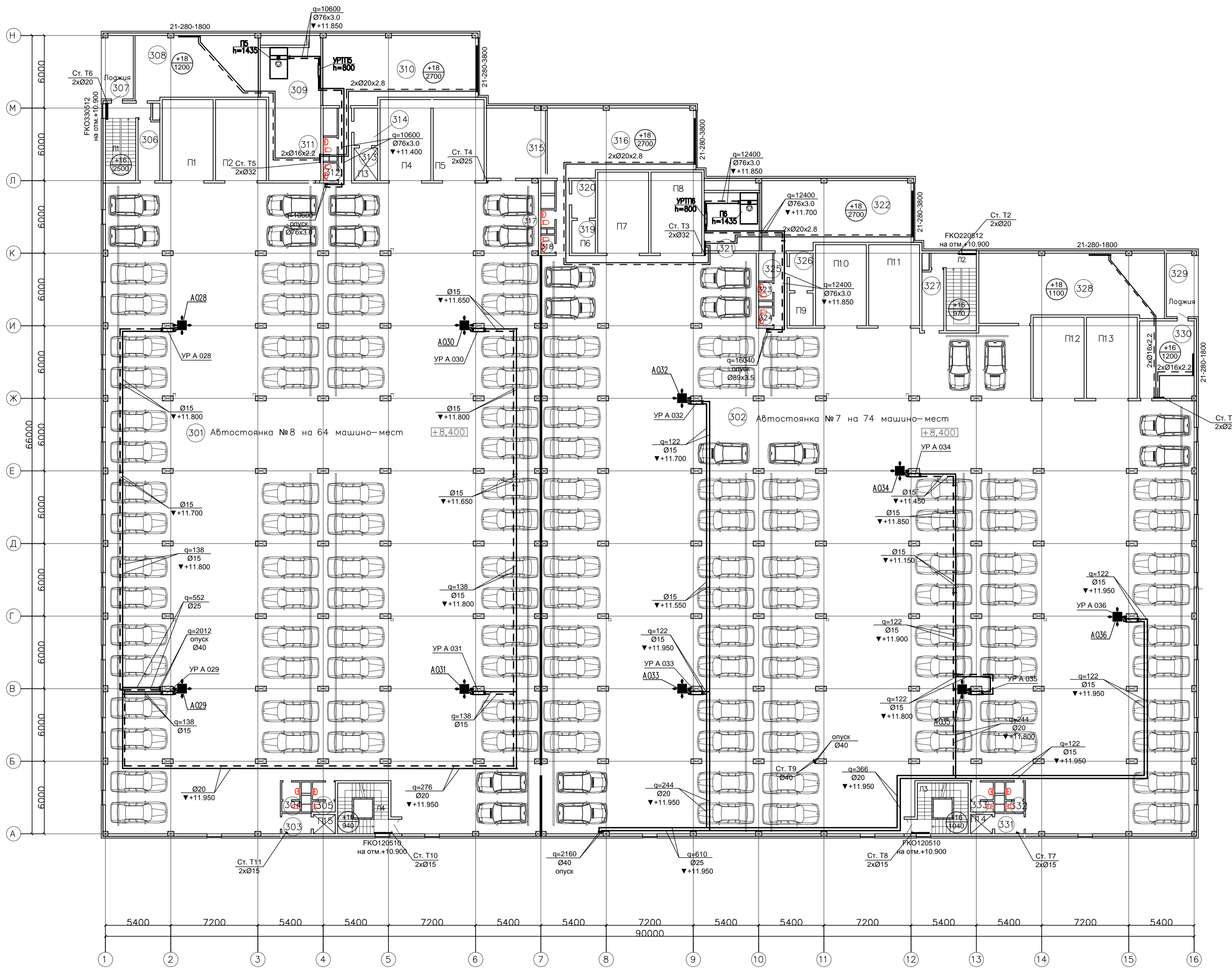
План 3-го этажа
