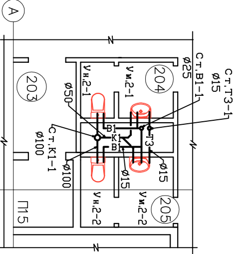
Фразмент плана в осях А-4 М 1:100
