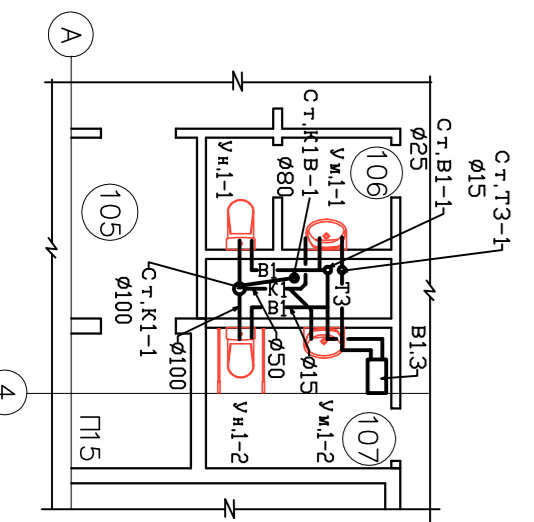
Фрагмент плана в осях А4 М 1:100
