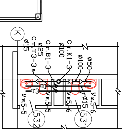
Фрагмент плана в осях К-7 М 1:100
